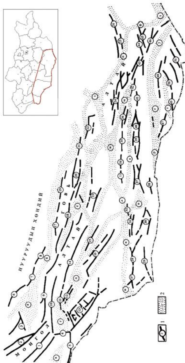
Зураг 4.14 Говь-Алтай ба Алтайн Өвөр говийн уул зүйн схем (Эх сурвалж: Тимофеев, Николаева, 1982, х. 87) 1-Уул нуруу: 1-Цагаанулуут уул, 2-Сутай уул, 3-Дарвийн нуруу, 4-Хөвчийн нуруу, 5-Тасхийн шар нуруу, 6-Хасагт Хайрхан уул, 7-Тайшарын нуруу, 8-Сэрх уул, 9-Буурал хайрхан, 10-Их талын нуруу, 11-Дан уул, 12-Торой нуруу, 13-Аж Богд, 14-Гичигийн нуруу, 15-Суман Хайрхан уул, 16-Эрэнгийн нуруу, 17-Хар Аргалант уул, 18-Баянцагаан уул, 19-Нарийн Хар уул, 20-22-Гурван Богд (20-Их Богд, 21-Бага Богд, 22-Ард Богд), 23-Шинэ Жинст, 24-Гурвансайхан, 25-Цэций уул, 26-Их Шанхай уул, 27-Агас Богд, 28-Чингис уул, 29-Булган Хушууны нуруу, 30-Цагаан Богд уул, 31-Цулуур хар нуруу, 32-Онгон-Шилийн уул, 33-Алтан уул, 34-Нэмэгт уул, 35-Сэрэйд уул, 36-Зөөлөн уул, 37-Тост уул, 38-Божууны толгой, 39-Хүрэн хаангийн нуруу, 40-Ноён уул, 41-Зурамгайн уул, 42-Их Аргалант, Бага Аргалант уул, 43-Номгон уул, 44-Ямаат уул, 45-Хаягч уул, 46-Хорх уул, 47-Сэрвэн Гүн-Элэн уул, 48-Баруун Цохионы нуруу, 49-Цагаан уул, 50-Хашаат уул, 51-Халзан уул, 2. Хотгорнууд: а-Шаргын говь, б-Выгэр, в-Зүүнгарын говь (Баруун Хуурай), г-Алаг нуур, д-Зах Борнуур, е-Баянцагаан, ж-Ширэг Гашуун, з-Улаан нуур, и-Номигийн говь, к-Алтайн өвөр говь, л-Ингэн Хөөвөр, м-Баяндалай, н-Хуцын Шанд, о-Гурван тэс, п-Даланзадгад, р-Галуун нуур, с-Бүгтийн хоолой, т-Улаан шал, у-Борлонгийн говь, ф-Баян-Овоо, х-Галбын говь.
